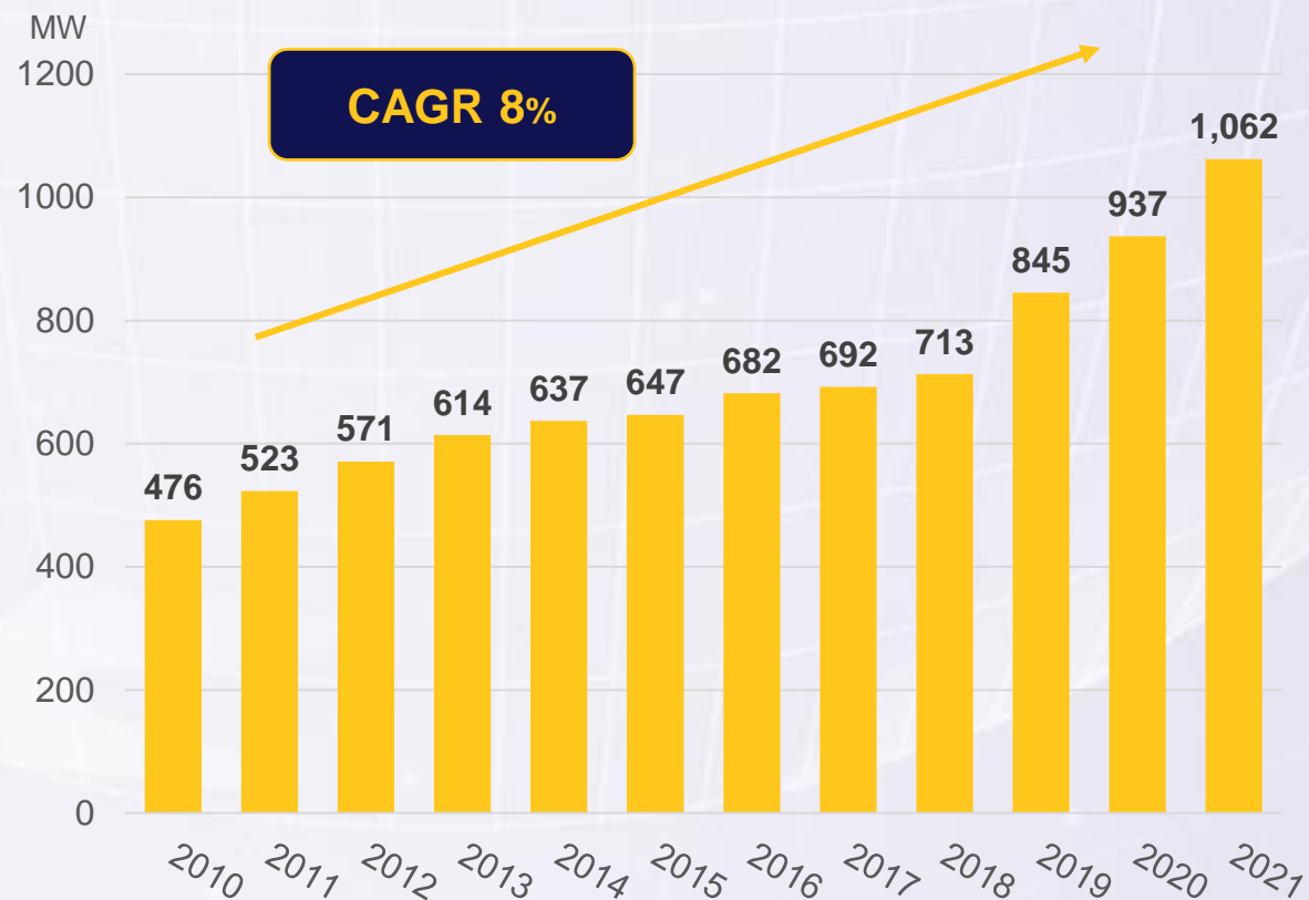
2010 – 2021年台灣風力發電容量建置概況
